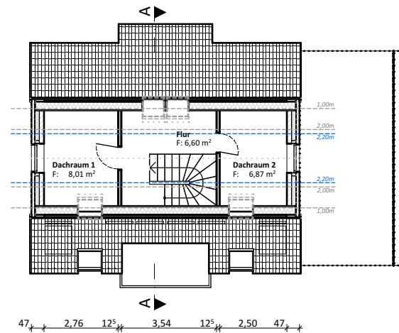
Grundriss Dachgeschoss
