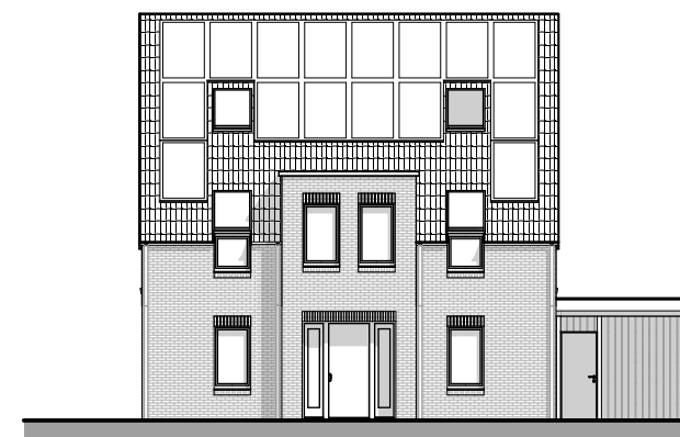
Ansicht Süd
