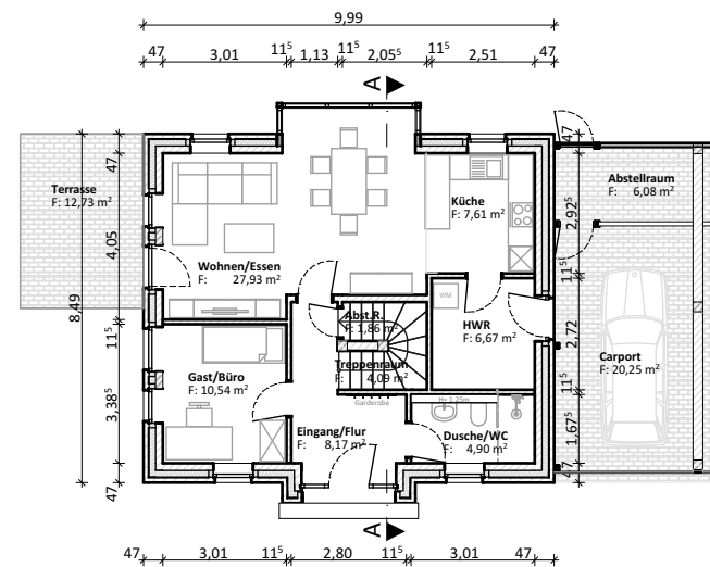
Grundriss Erdgeschoss
