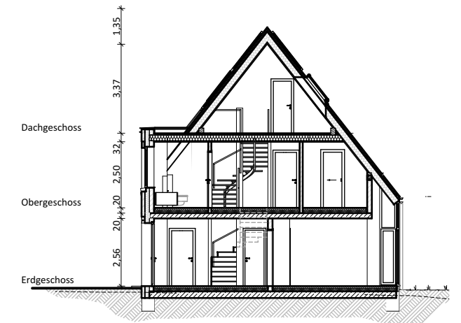
Schnitt A-A
