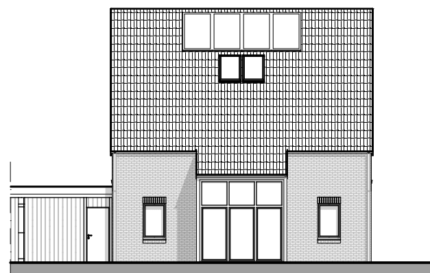
Ansicht Nord
