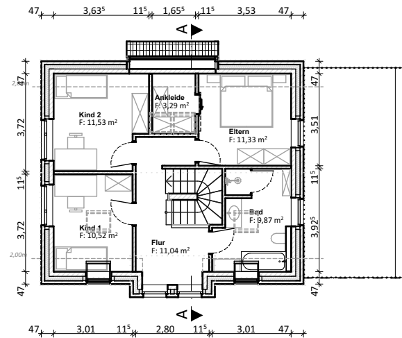
Grundriss Obergeschoss
