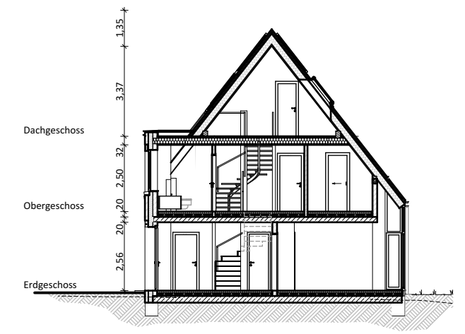
Schnitt A-A
