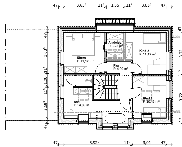
Grundriss Obergeschoss
