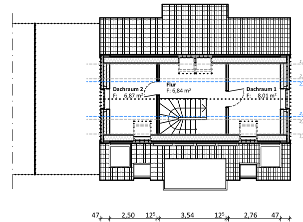
Grundriss Dachgeschoss
